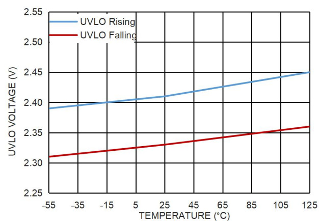
图 13. UVLO 阈值
