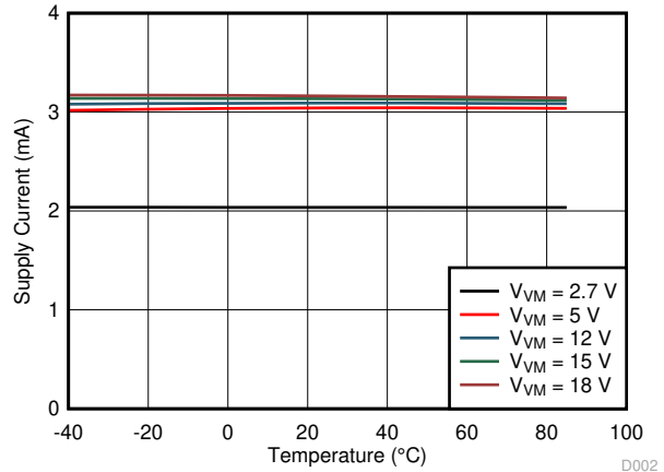
图 6-4. 工作电源电流 ( I_{VM} ) 与环境温度 ( T_A ) 间的关系
