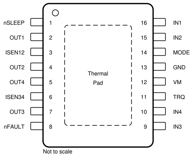
图 5-2. DRV8847 PWP PowerPAD™ 封装 16 引脚 HTSSOP 顶视图
