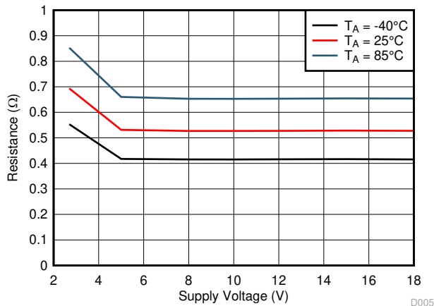
图 6-7. 高侧导通状态电阻 ( R_{DS(ON)_HS} ) 与电源电压 ( V_{VM} ) 间的关系
