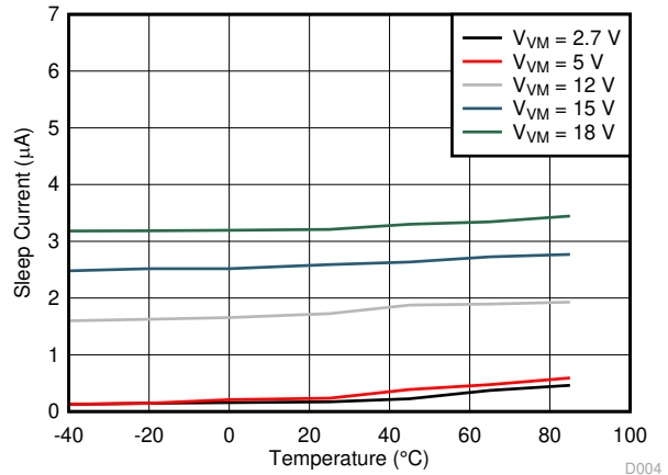
图 6-6. 睡眠模式电源电流 ( I_{VMQ} ) 与环境温度 ( T_A ) 间的关系
