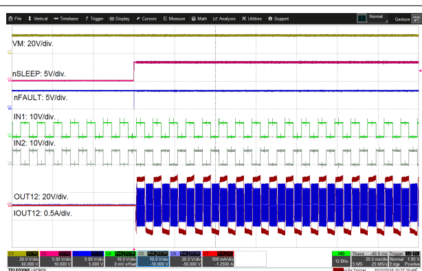
图 8-6. 通过 nSLEEP 引脚实现器件上电
