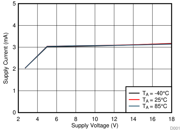
图 6-3. 工作电源电流 ( I_{VM} ) 与电源电压 ( V_{VM} ) 间的关系
