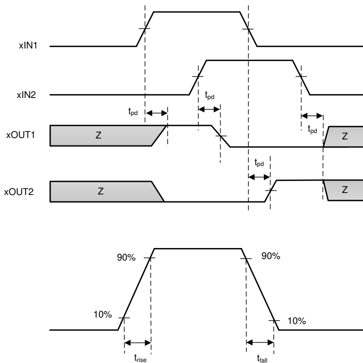
图 6-1. 时序图
