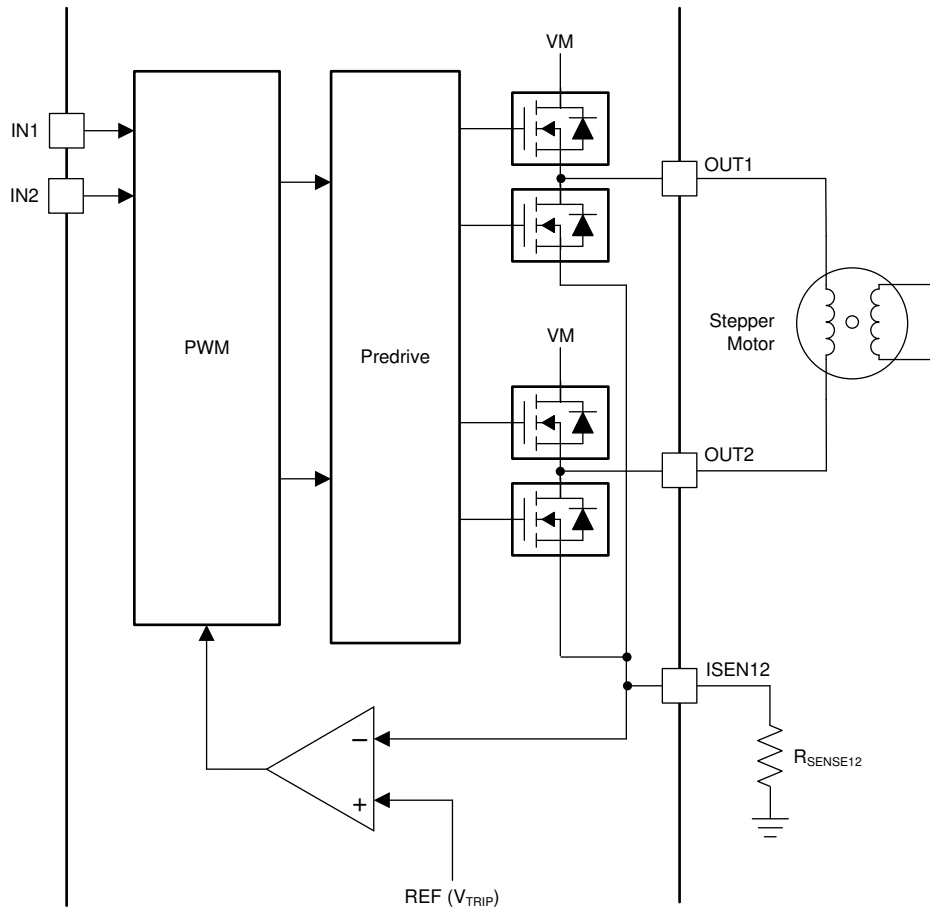
图 7-3. PWM 电机驱动器电路
