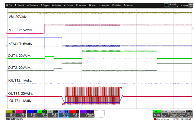
图 8-14. 开路负载检测操作
