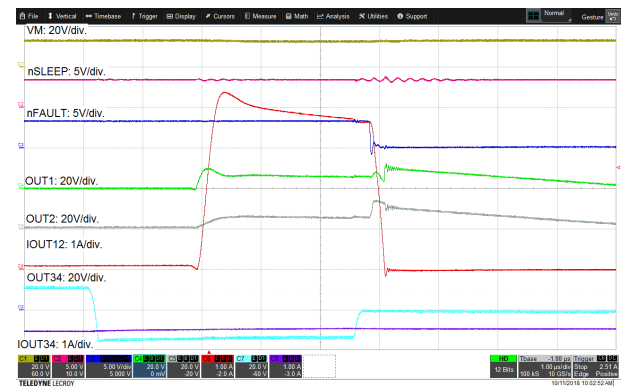
图 8-16. 过流保护放大波形
