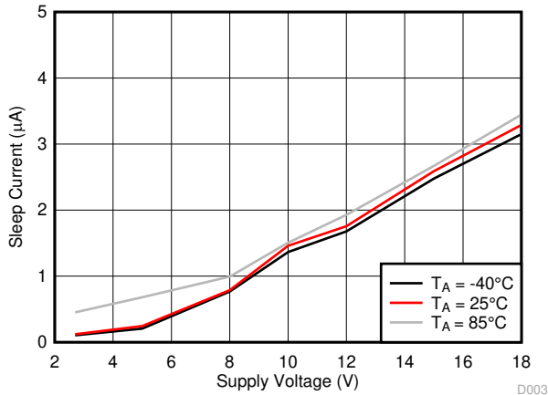
图 6-5. 睡眠模式电源电流 ( I_{VMQ} ) 与电源电压 ( V_{VM} ) 间的关系
