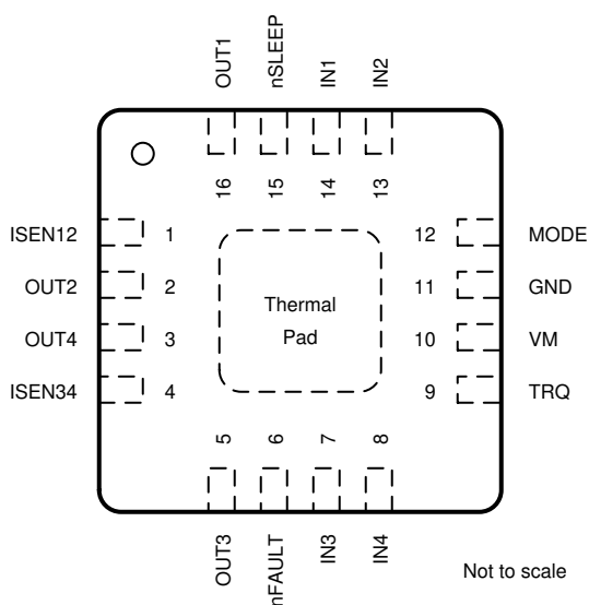
图 5-3. DRV8847 RTE 封装 16 引脚 WQFN (带有外露散热焊盘) 俯视图
