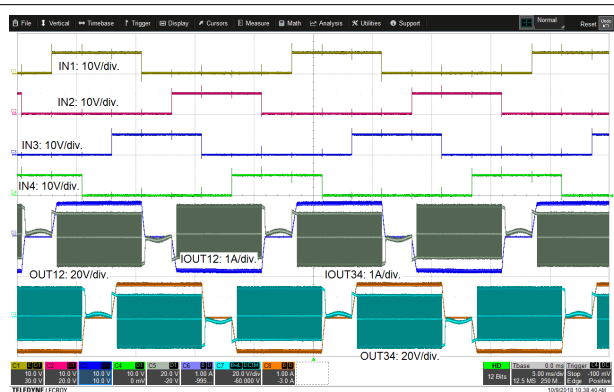
图 8-8. 关断状态高阻态模式下的步进电机半步运行
