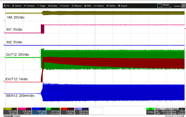
图 8-10. 并联模式下的有刷直流电机运行，显示 2A 时的电流调节
