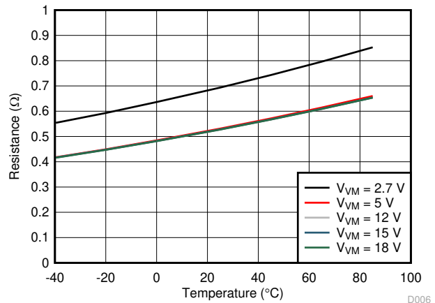
图 6-8. 高侧导通状态电阻 ( R_{DS(ON)_HS} ) 与环境温度 ( T_A ) 间的关系
