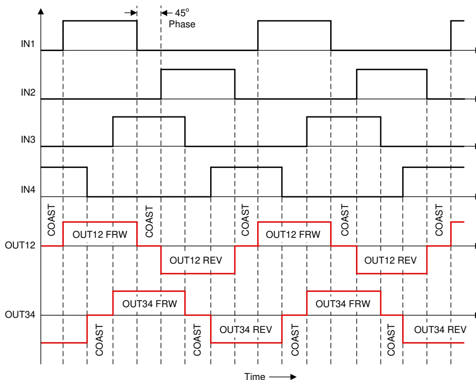
图 7-16. 使用 4 引脚连接的半步进模式（非驱动快速衰减）
