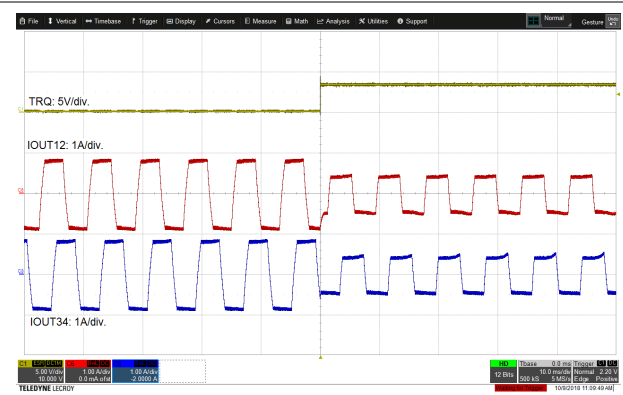
图 8-12. 用于调节电流的扭矩引脚功能
