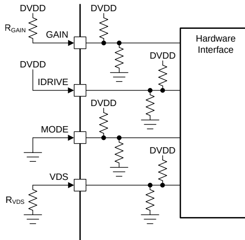
图 18. Hardware Interface
