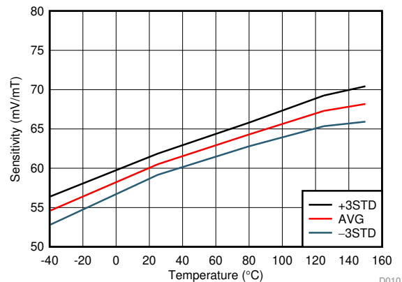
图 5-8. 灵敏度与温度之间的关系
