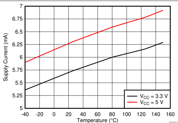
图 5-1. 电源电流与温度间的关系
