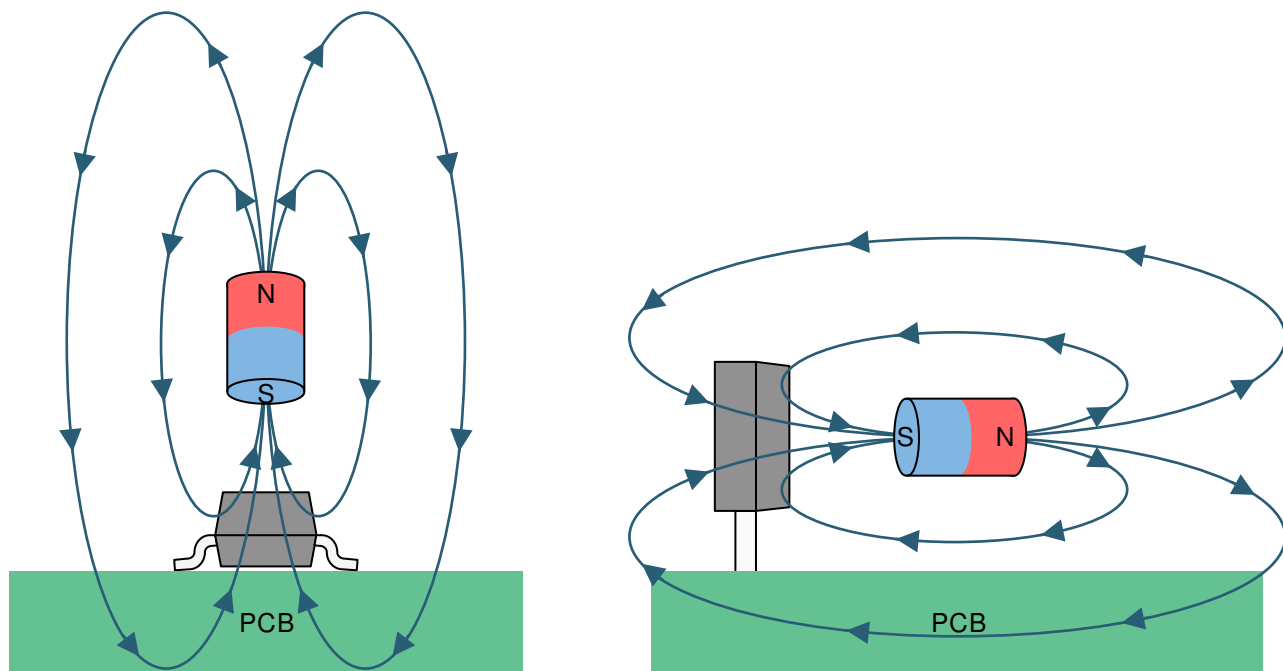
图 6-2. 正 B 的磁通方向
