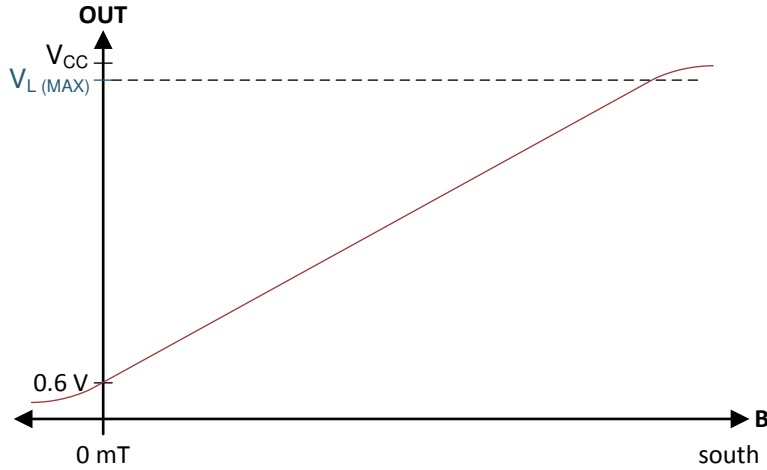
图 6-3. 磁响应
