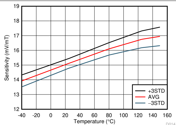
图 5-10. 灵敏度与温度之间的关系
