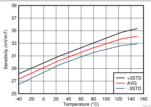
图 5-8. 灵敏度与温度之间的关系
