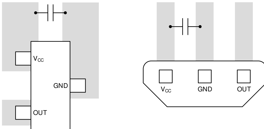
图 7-6. 布局示例
