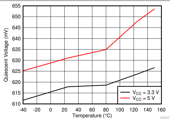
图 5-3. 静态电压与温度之间的关系
