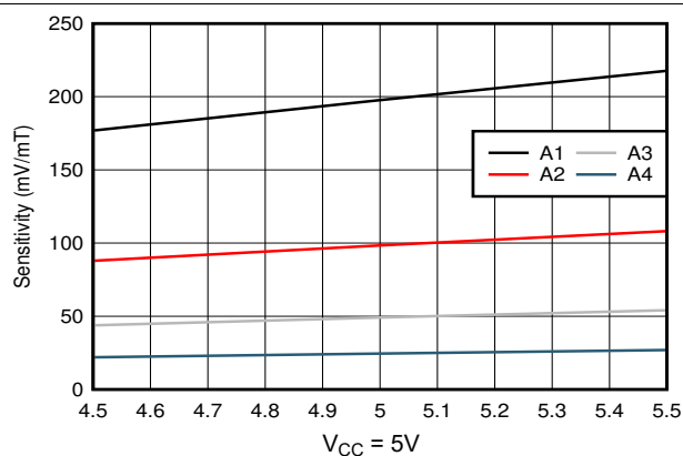
图 5-5. 灵敏度与电源电压之间的关系
