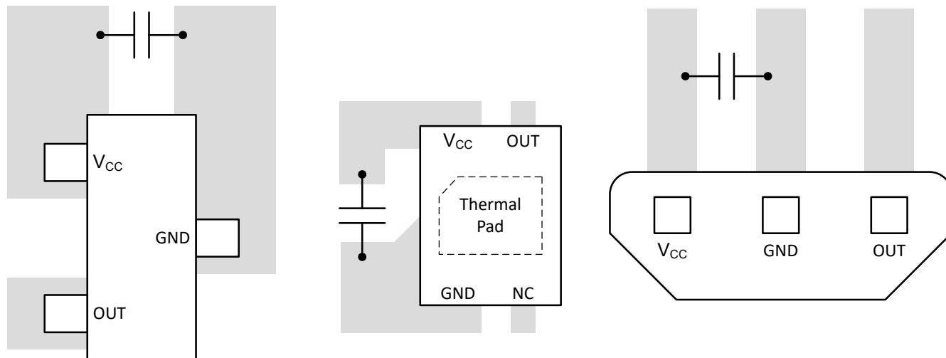
图 8-7. 布局示例
