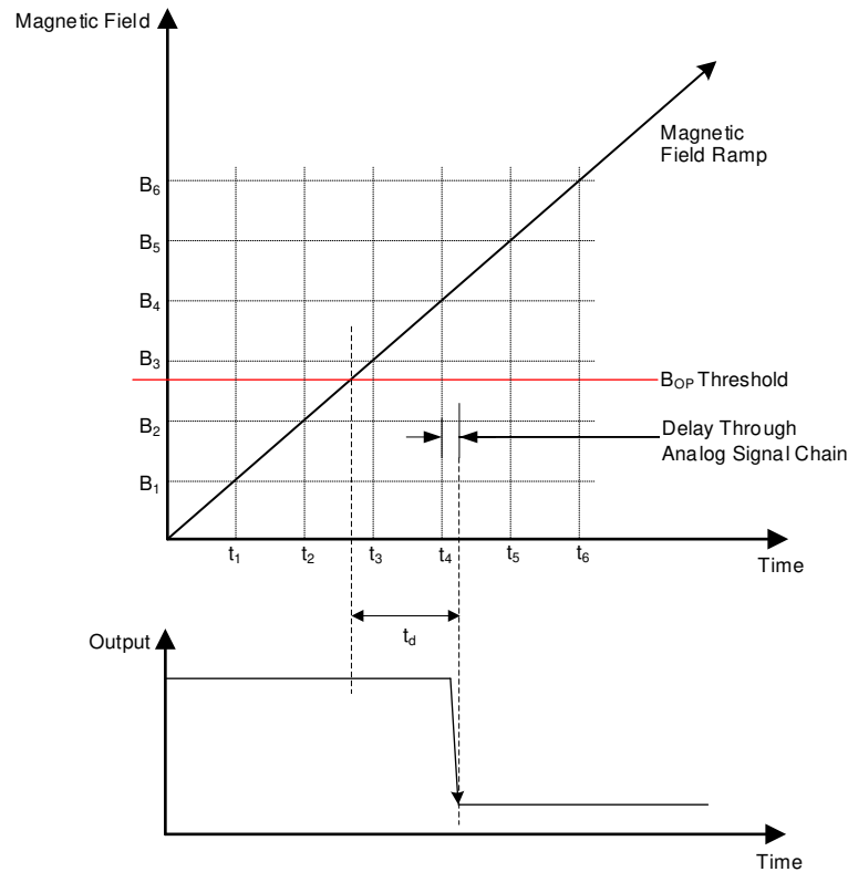
图 18. Propagation Delay
