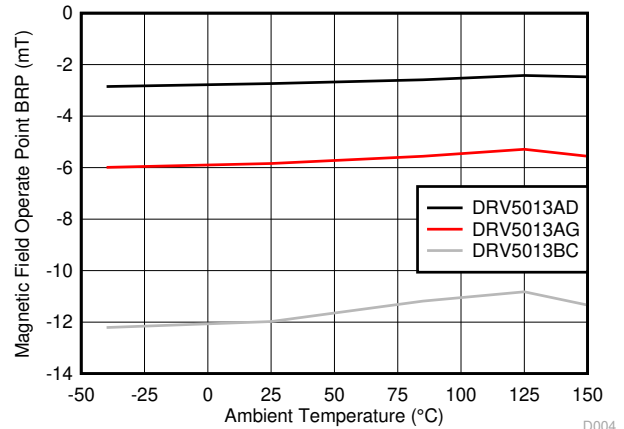
图 6-4. B_{OP} 与温度之间的关系
