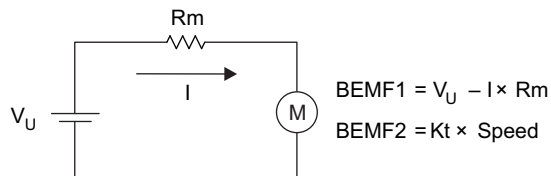
图 30. Lock Detection 1
