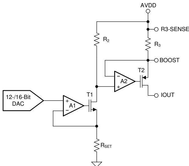
图 8-2. Current Output
