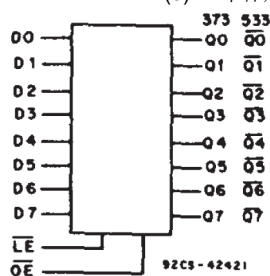
逻辑图 (正逻辑)
