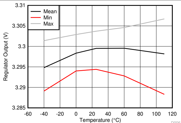
图 6-6. 无负载时的稳压器输出
