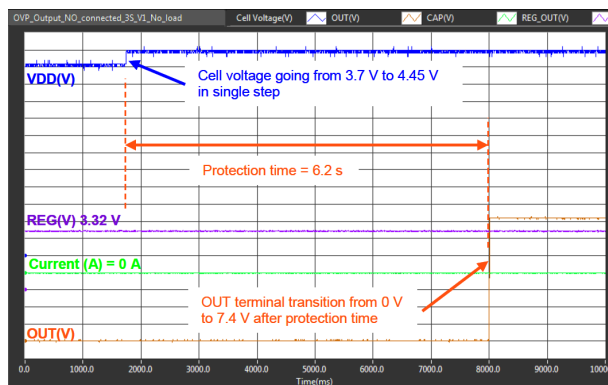
图 8-4. 过压保护
