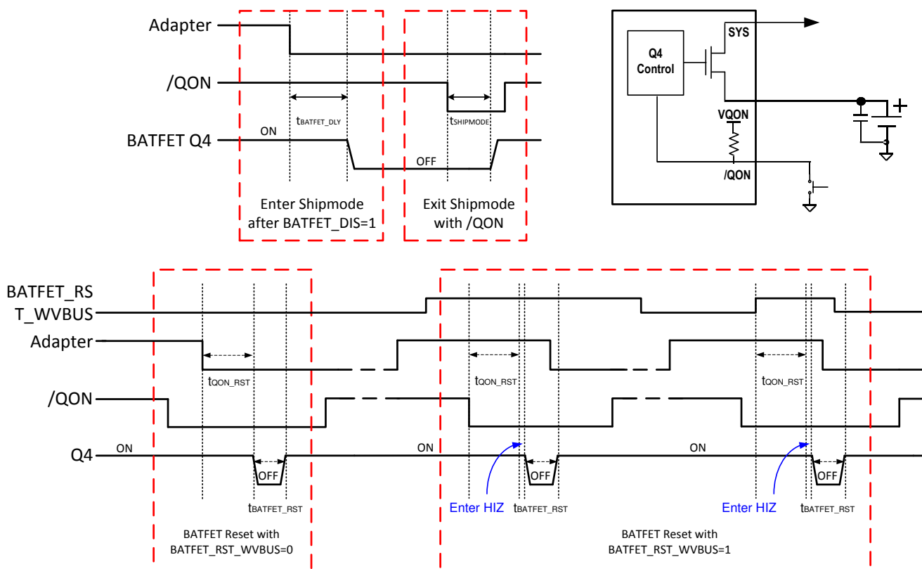
图 7-6. QON Timing
