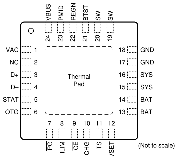
图 7-1. BQ25606 RGE Package 24-Pin VQFN Top View
