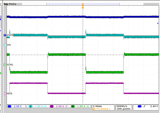
图 10-11. OTG Switching
