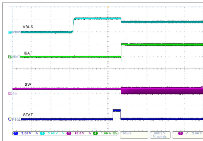
图 10-6. VBUS startup into VINDPM
