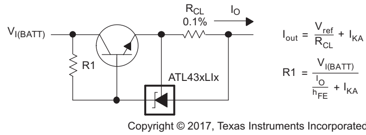
图 39. 精密限流器
