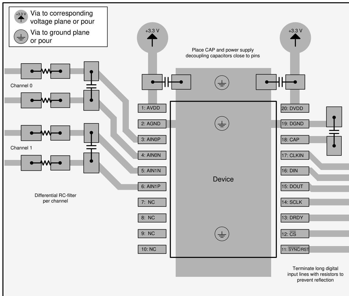
图 11-1. Layout Example
